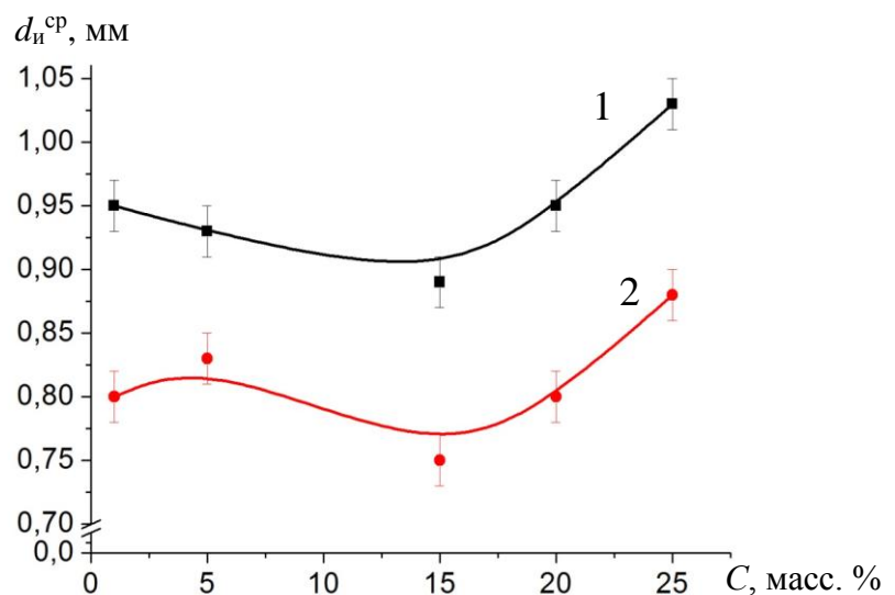
1 – при нагрузке 40 кг; 2 – при нагрузке 20 кг Рисунок 2. – Зависимость диаметра пятна износа ( d_{и}^{сп} ) шаров от содержания графита в смазочном материале
