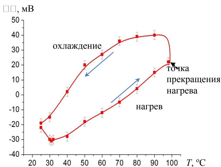
Рисунок 3. – Зависимость разности потенциалов от температуры электродов (ст. 50) в 0,1н растворе NaCl
