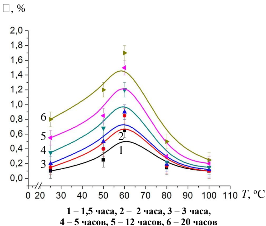
Рисунок 4. – Интенсивность процесса синерезиса, в зависимости от температуры и времени эксплуатации композиционного материала
